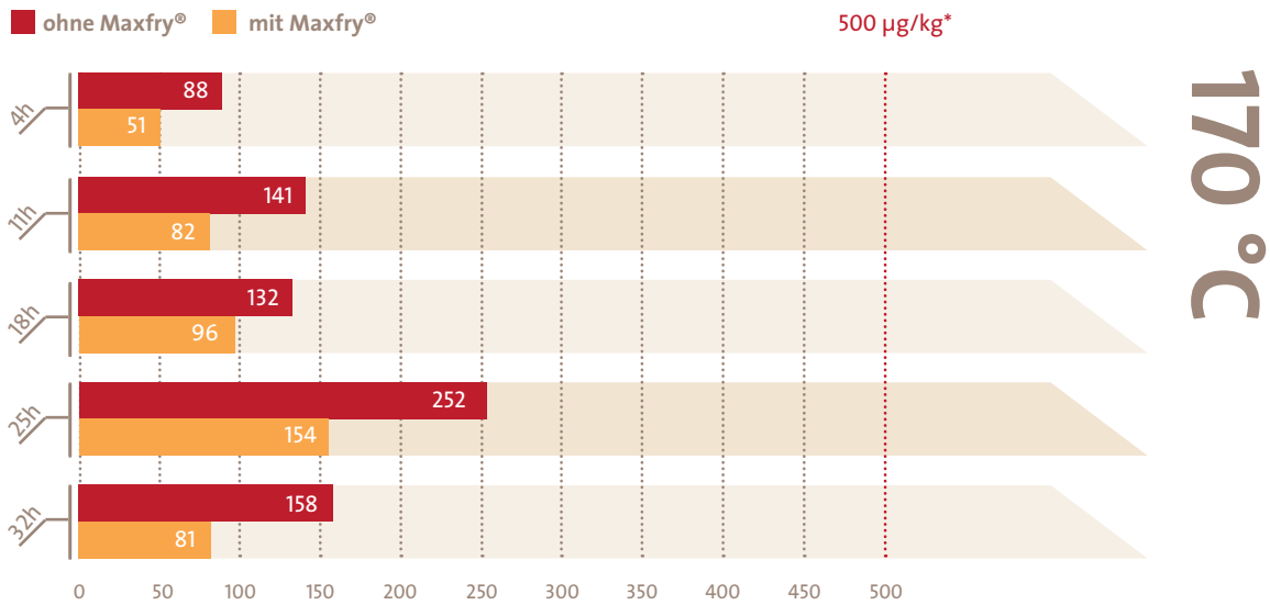
Bildung von Acrylamid (µg/kg) in Pommes frites frittiert in Rapsöl mit und ohne Maxfry® bei 170 °C/180 °C
